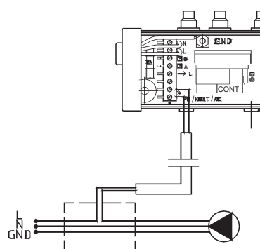
Anschluß der Pumpe bei Kontaktausgang
