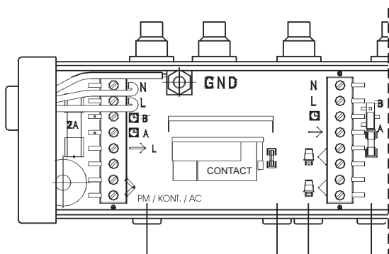
Pumpenabschaltmodul ZRP mit Kontaktausgang für die Pumpe
